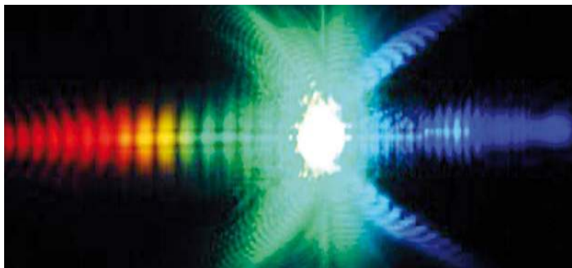
Abb. 5) Aufnahme einer „konischen Welle“ aus dem Bereich der nicht-linearen Optik
