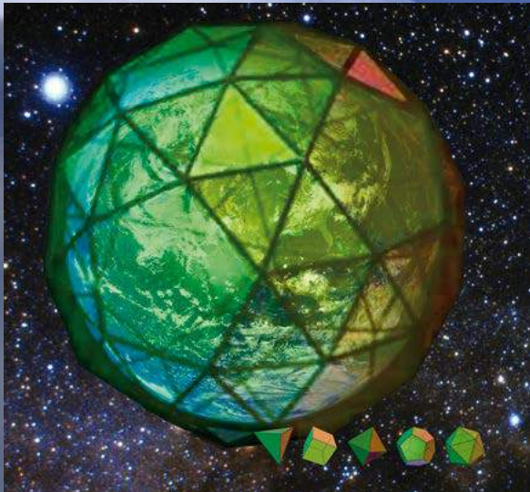
Abb. 1) Schwingungen, die um die Erde laufen, sind stabil, wenn sie nach einem Umlauf wieder harmonisch an sich selber anschließen. Auf einer Kugeloberfläche gibt es hierzu eine begrenzte Anzahl mathematischer Lösungen, die sich durch die Platonischen Körper darstellen lassen. Auf den Kanten der platonischen Körper liegen die Schwingungsknoten, auf den Flächen die Schwingungsbäuche. Alle fünf Platonischen Körper sind in dieser Form in dem Schwingungsfeld der Erde manifestiert.
